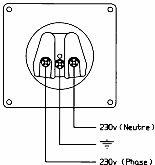
PLAN DE CABLAGE
