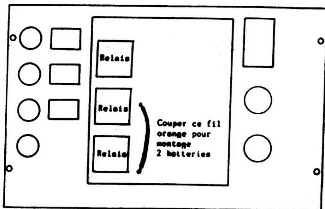
VUE ARRIERE DE L'ALIMENTATION
